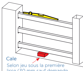
2 - Positionner la trame et caler
