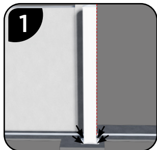
1 Positionner le poteau pour l'aligner au pilier et tracer les repères
