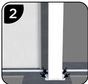
2 Fixer le poteau. Nous préconisons l'utilisation de tiges filetées avec scellement chimique : - Ø 10 mm pour poteau 150x150 mm - Ø 12 mm pour poteau 188x188mm
