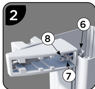
Glisser le boulon dans la rainure pour fixer.
