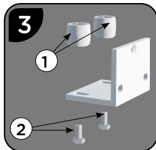
3 Monter les olives de guidage
