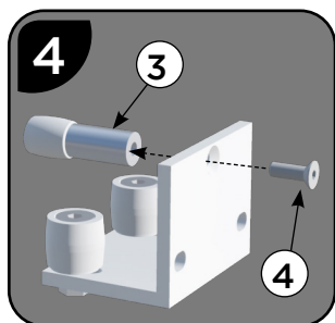
4 Monter le doigt de guidage
