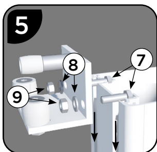
5 Glisser les boulons dans les rainures puis fixer provisoirement le support.
