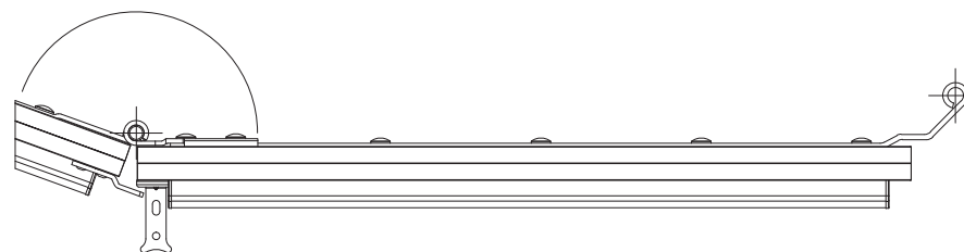
Dardennes alignées au Vantail Porteur
