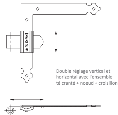
Équerre aluminium réglable réversible feston 34x4 trous carrés
