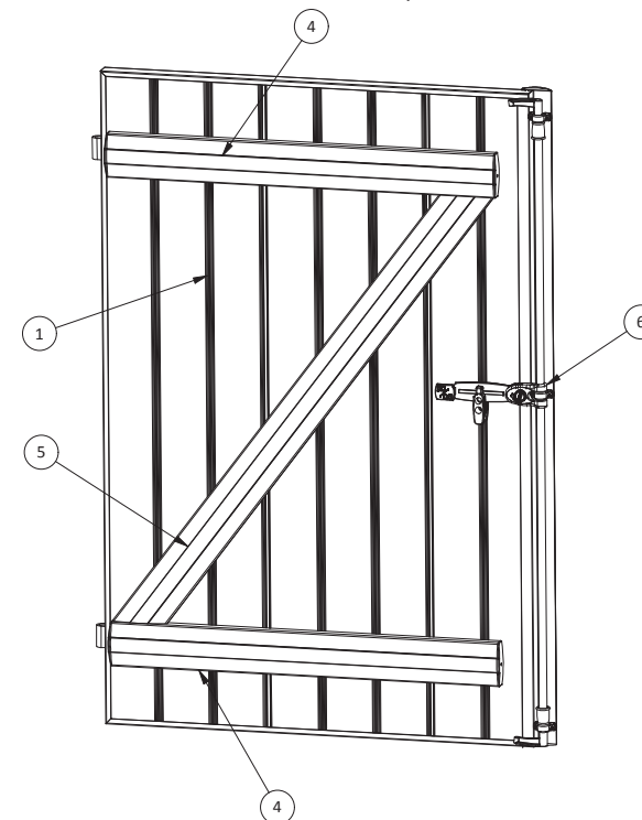
VB - Barre écharpe
