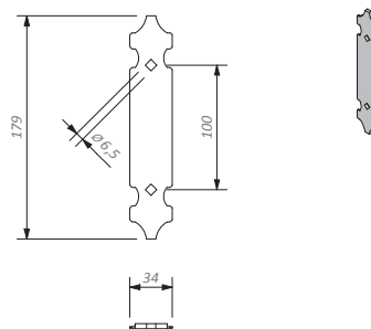
Té alu réglable réversible feston 34x4 trous carrés L179
