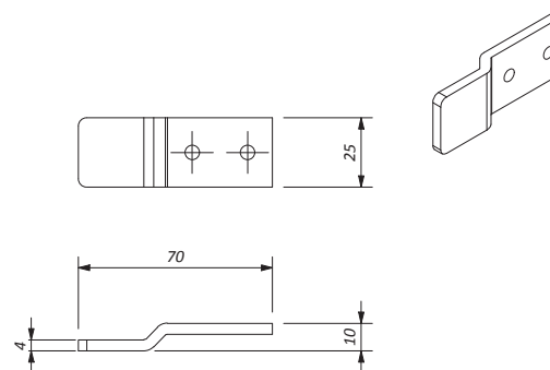
Crochet de rappel VT repliable en fourniture avec rivets 4,8x16 Ref. 4158
