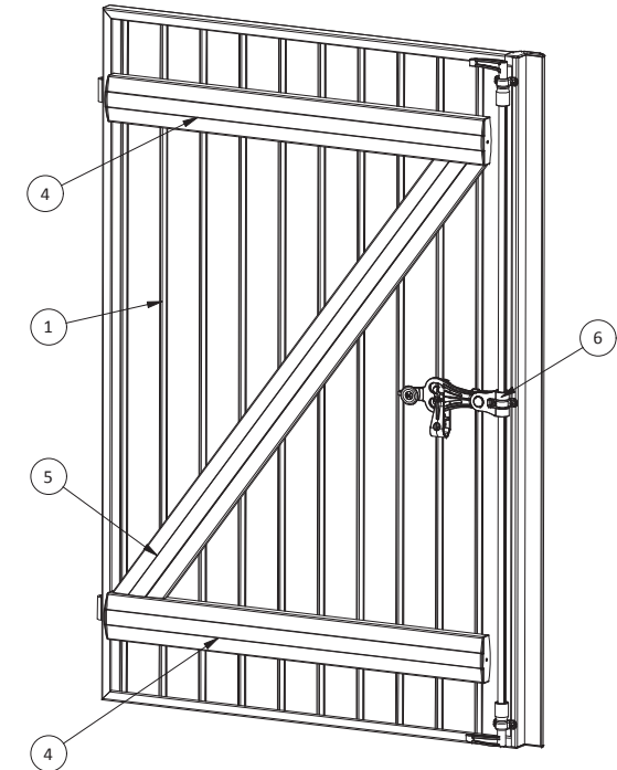
VB - Barre écharpe
