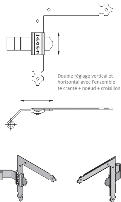
Equerre aluminium réglable réversible feston 34x4 trous carrés
