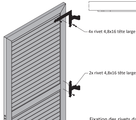
Fixation des rivets dans les renforts (pour Cadre PVC soudé)
