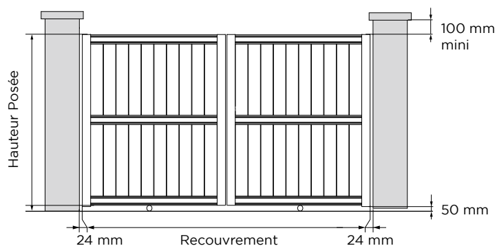
COULISSANT
