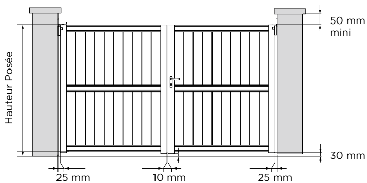
BATTANT
