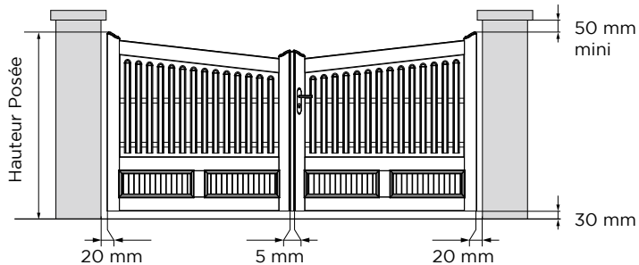
BATTANT
