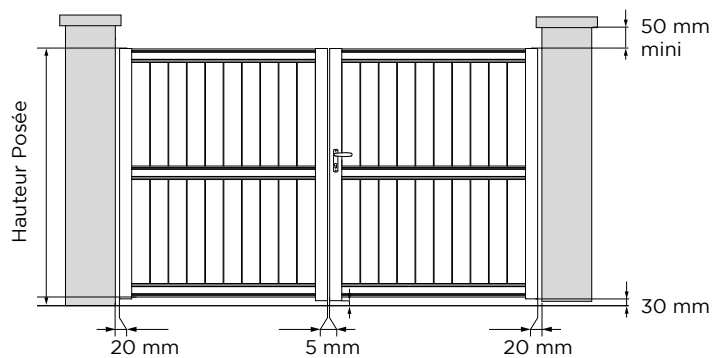
BATTANT
