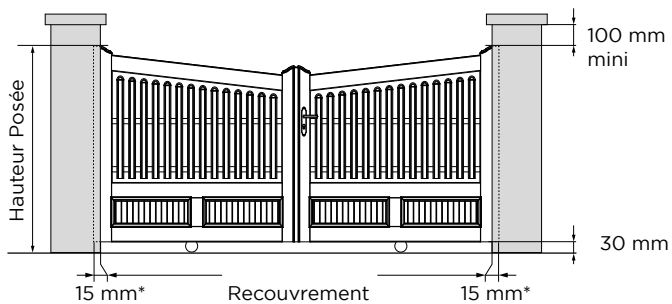
COULISSANT
