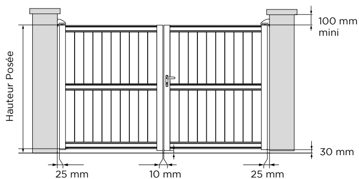
BATTANT
